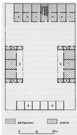
Pianta tipo cascina ad elementi separati
