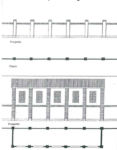
Rustico storico posto lungo il muro di recinzione
