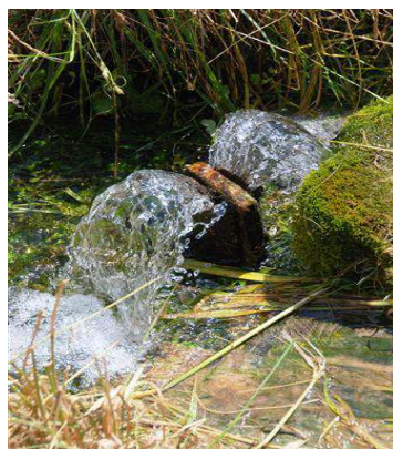
Fontanile a Cremona (CR); sono evidenti l'occhio (o polla) nella testa del fontanile, la palificata di contenimento spinale e la vegetazione igrofila lungo l'asta
